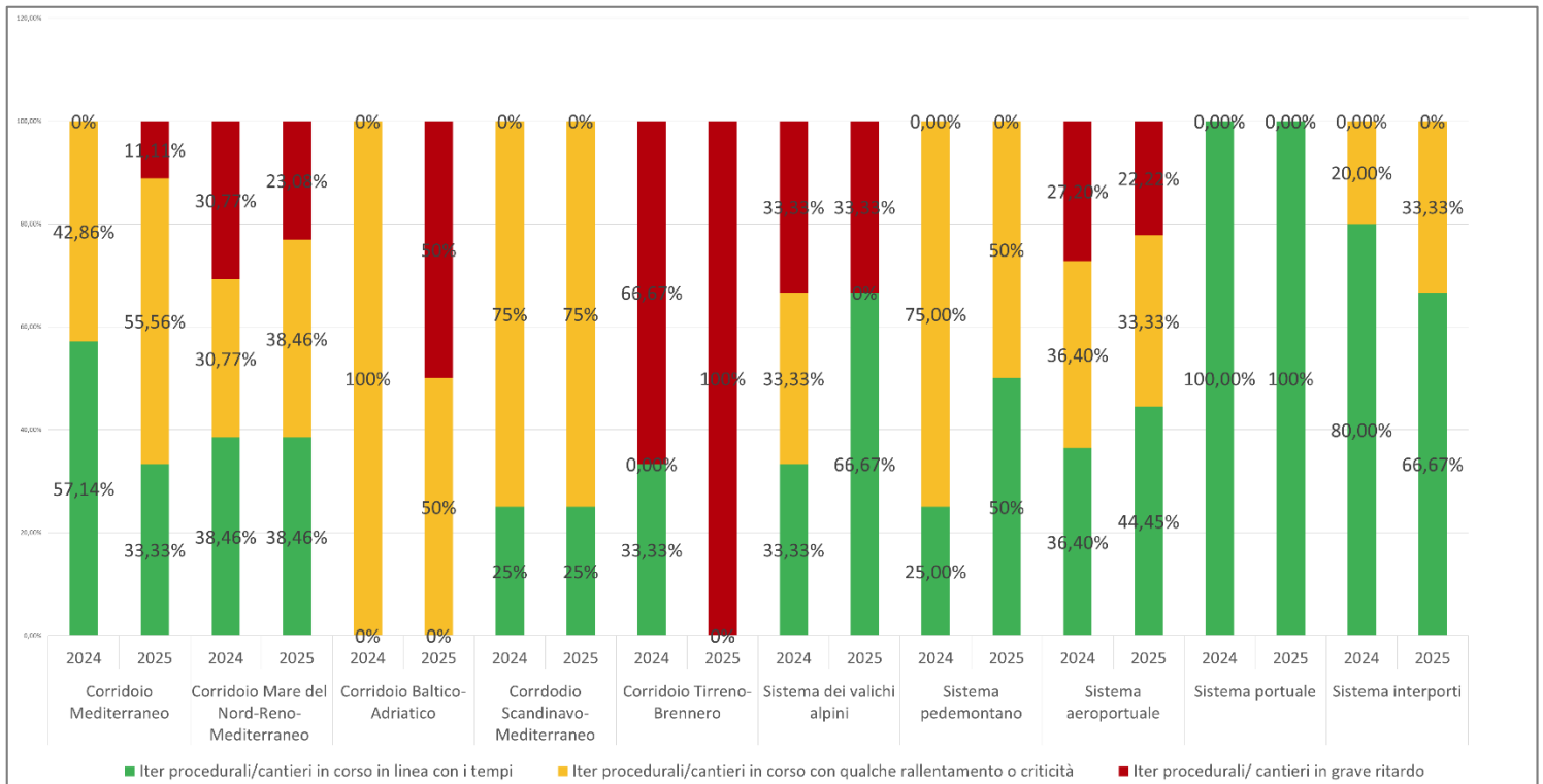
GRAFICO 2A – STATO DI AVANZAMENTO OPERE PER SISTEMI INFRASTRUTTURALI (esclusi i Nodi metropolitani). CONFRONTO 2024-2025
